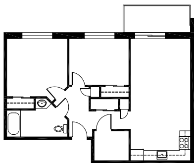
Logement type B - 2cc 70 m 2
