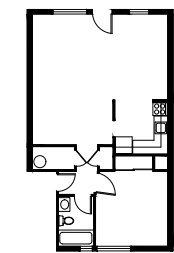
Rez-de-chaussée Logement type A - 1cc 57 m 2
