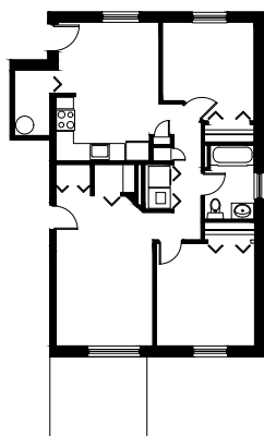
Logement type B - 2cc 71 m 2
